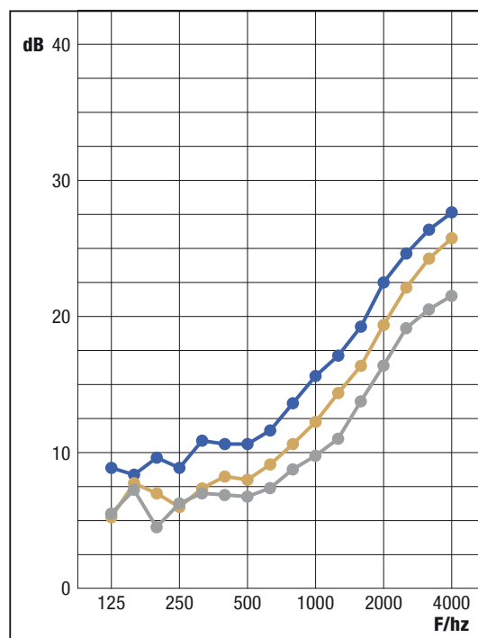
Schalldämm-Maße / Indices d'affaiblissement acoustique / Sound reduction factor
