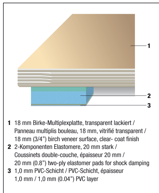
Bodenaufbau / Construction du tapis / Floor Composition
